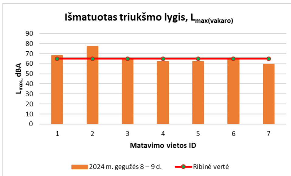
35 pav. Maksimalaus triukšmo pasiskirstymas matavimo vietose vakaro metu (19-22 val.). Ribinis dydis 65 dBA.
