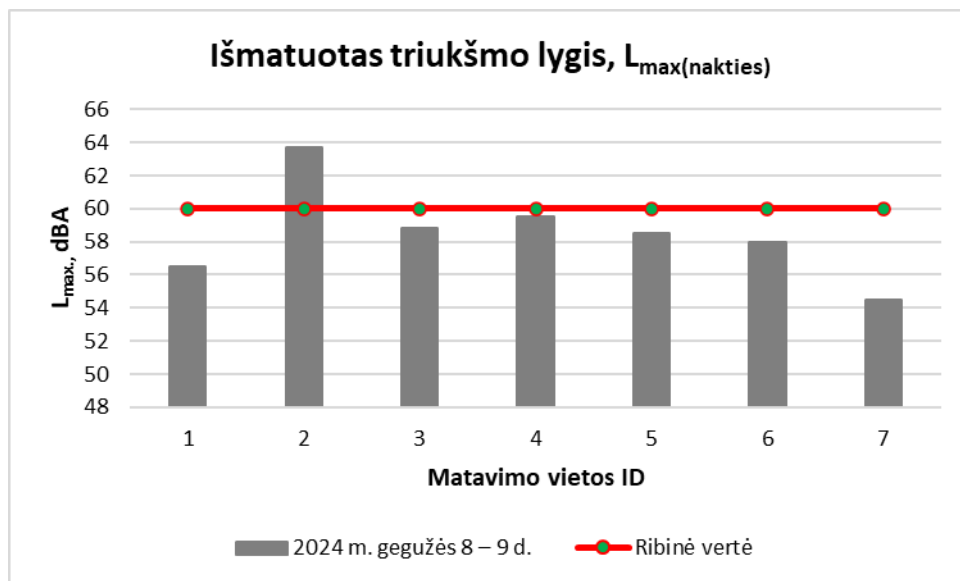
37 pav. Maksimalaus triukšmo pasiskirstymas matavimo vietose nakties metu (22-7 val.). Ribinis dydis 60 dBA.
