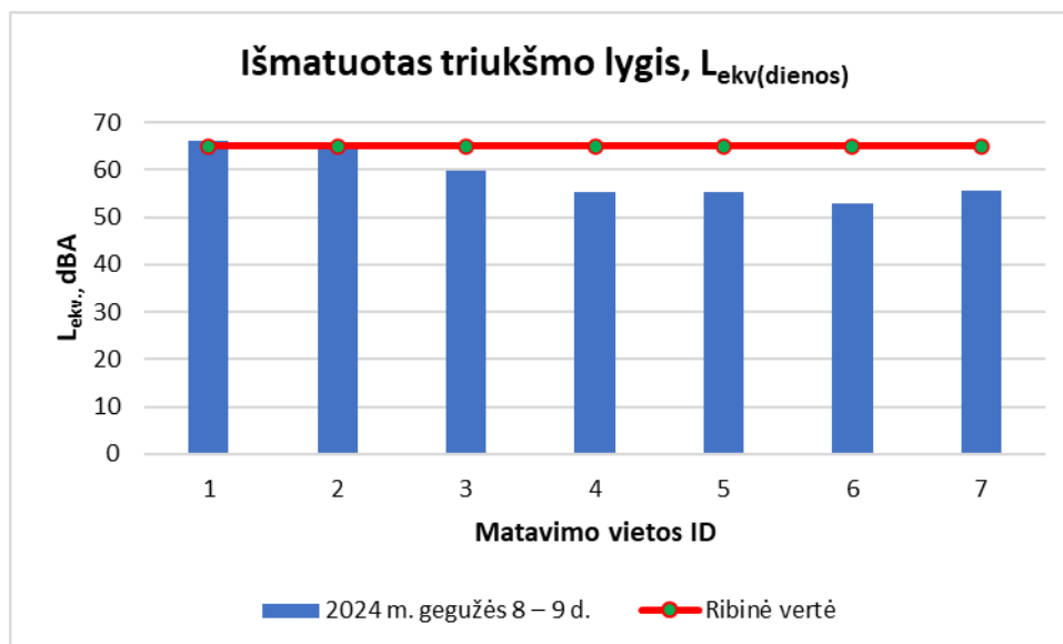
34 pav. Ekvivalentinio triukšmo pasiskirstymas matavimo vietose dienos metu (7-19 val.). Ribinis dydis 65 dBA.
