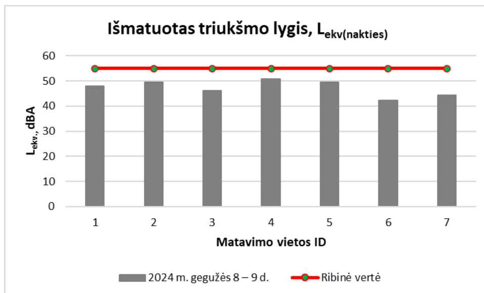
38 pav. Ekvivalentinio triukšmo pasiskirstymas matavimo vietose nakties metu (22-7 val.). Ribinis dydis 55 dBA.
