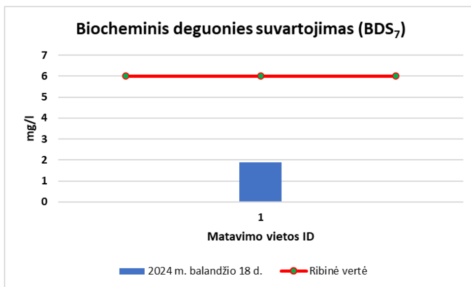
26 pav. BDS 7 verčių pasiskirstymas ežere, Zarasų rajone, nustatytoje matavimo vietoje
