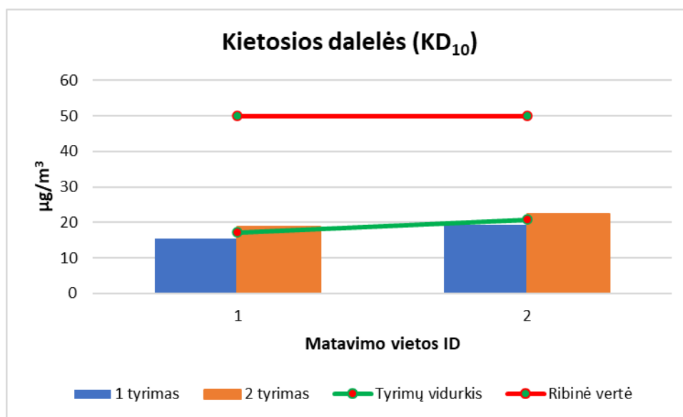
11 pav. KD 10 koncentracijų pasiskirstymas Zarasų rajone, nustatytose matavimų vietose
