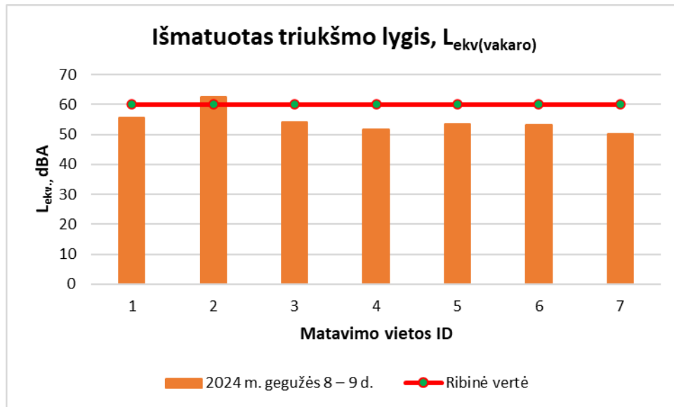
36 pav. Ekvivalentinio triukšmo pasiskirstymas matavimo vietose vakaro metu (19-22 val.). Ribinis dydis 60 dBA.
