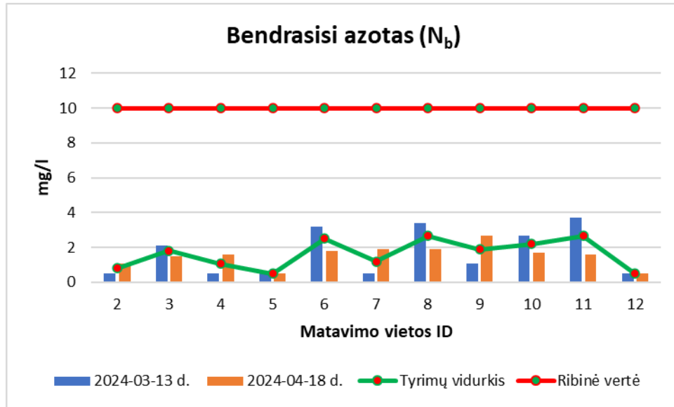
17 pav. Zarasų rajono savivaldybės upių vandens N bendrojo tyrimo rezultatų vizualizacija
